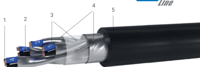
1. Rame rosso o stagnato Classe 1 o 2 o 5 | Tinned or bare copper Class 1 or 2 or 5 • 2. PVC • 3. Nastro di poliestere | Polyester tape • 4. Schermo a nastro di alluminio/poliestere con conduttore di drenaggio in rame stagnato | Aluminium | Polyester tape screen with tinned copper drain wire • 5. PVC
